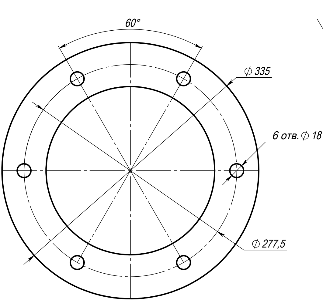
25.SHT.G.04.00.00.01 Фланец 2 шт.
