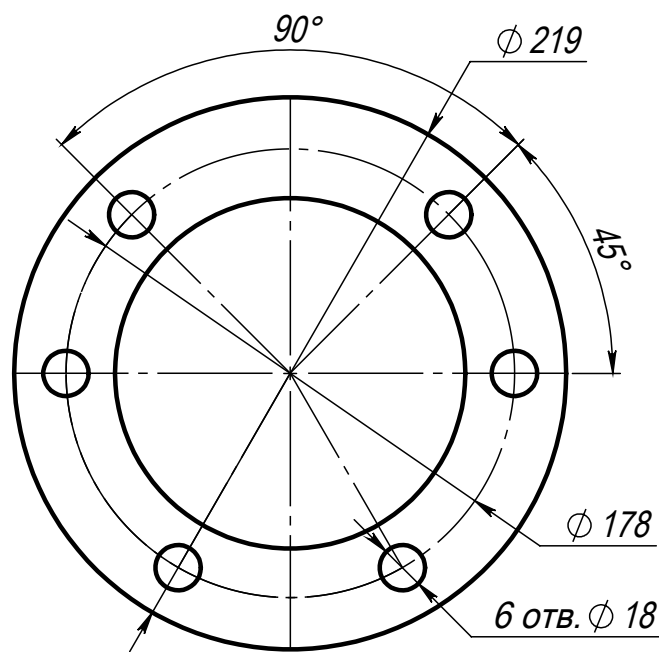
25.SHT.G.05.00.00.02 Фланец редуктора 1 шт.
