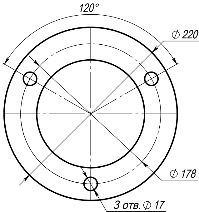
25.SHT.G.03.00.00.02 Фланец 1 шт.
